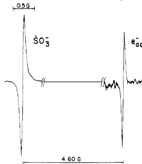
Спектр ЭПР e^-_{aq} при 296 K (Jeevarandan & Fessenden J. Phys. Chem., 1989, 93 , 3511) – in situ фотолит сульфита Спектры не зависят от метода генерации
